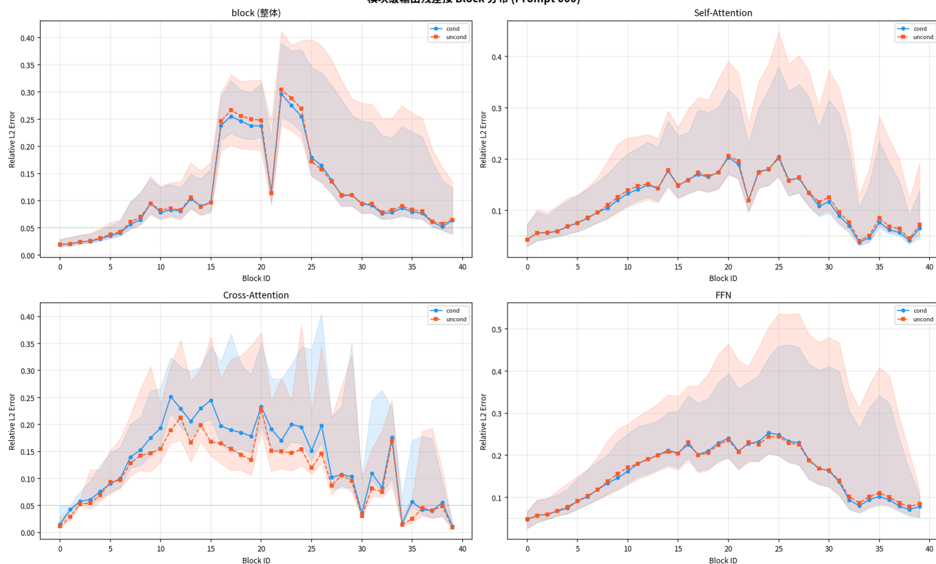
模块级输出残差按 Block 分布 (Prompt 000)
