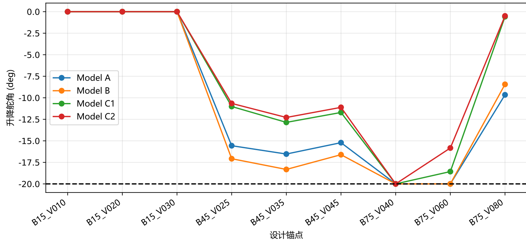
升降舵角对比
