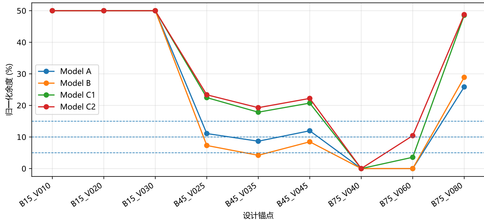
升降舵余度与假设设计阈值
