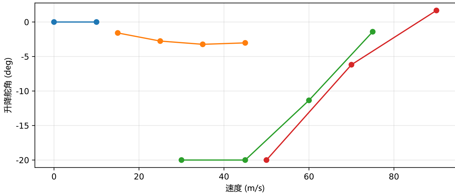
密集网格升降舵曲线
