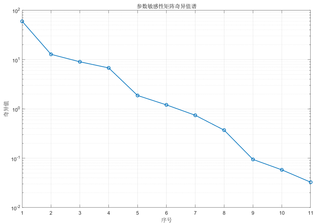
图 9.9 参数敏感性矩阵的奇异值分解
