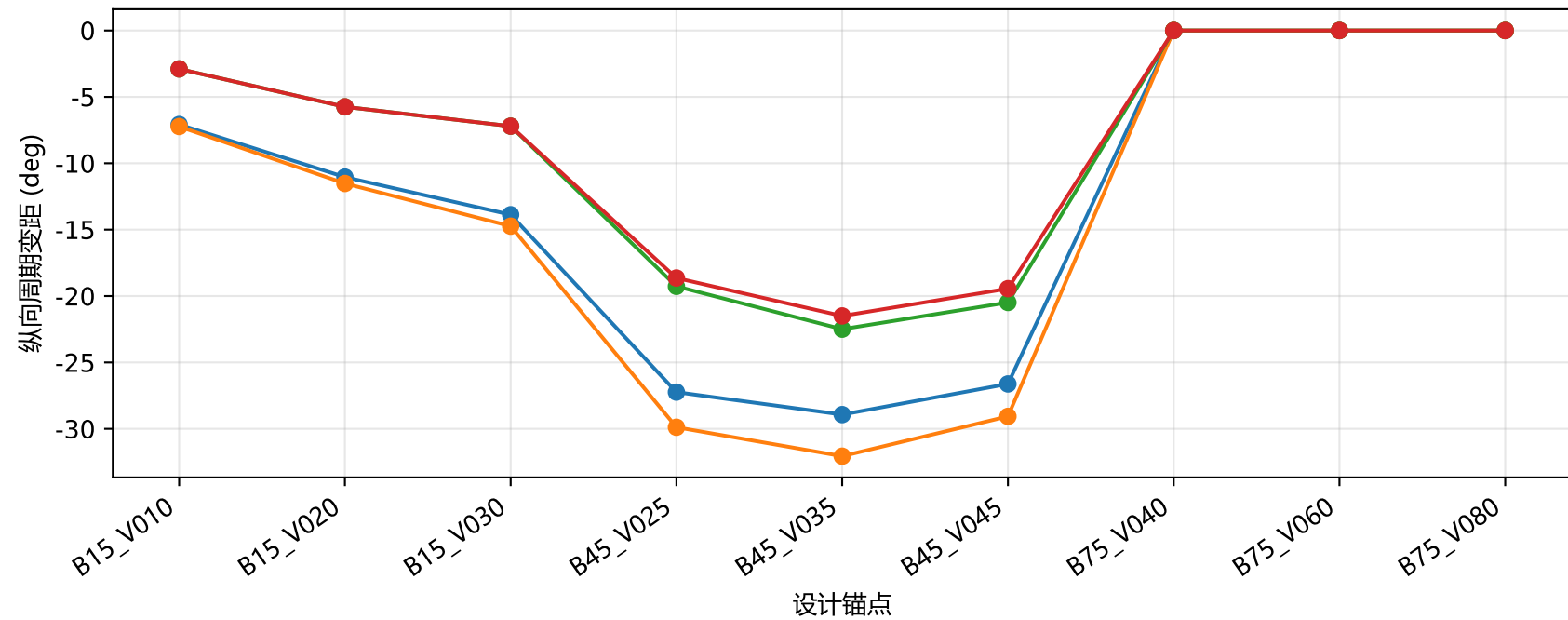
纵向周期变距对比
