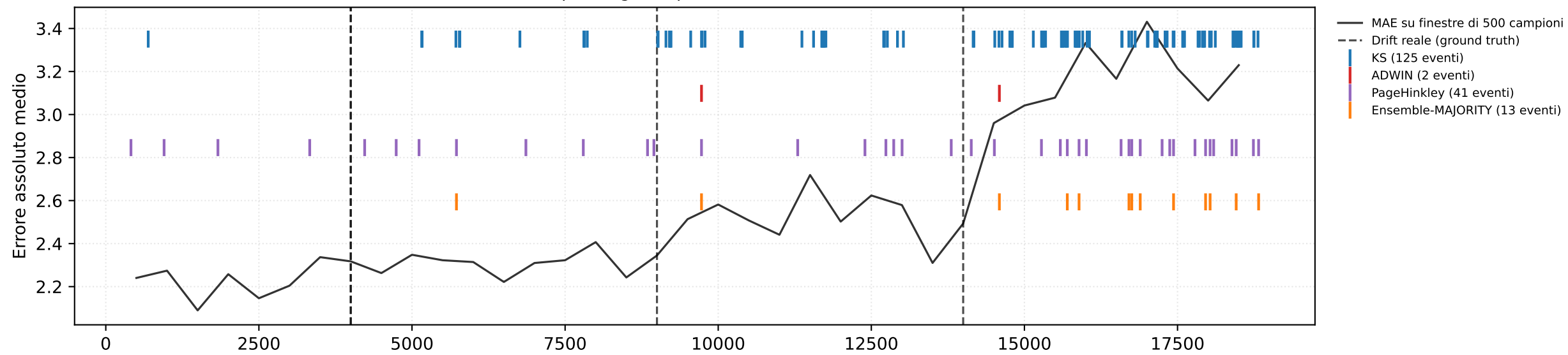
gra — Global Recurring Abrupt drift (il concetto iniziale ritorna)
