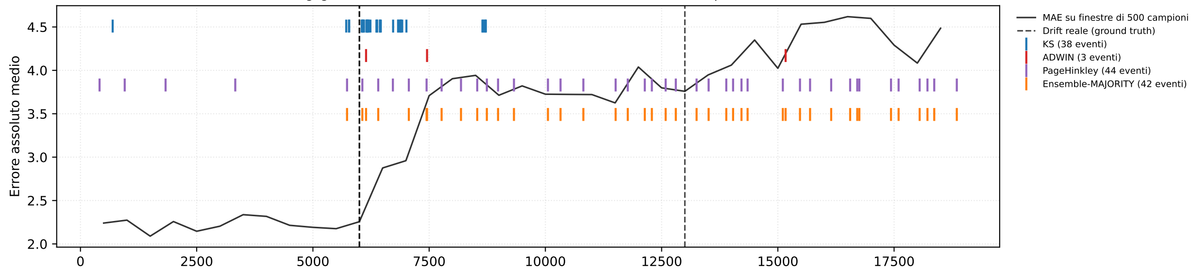
gsg — Global Slow Gradual drift (transizione lenta di 1000 campioni)
