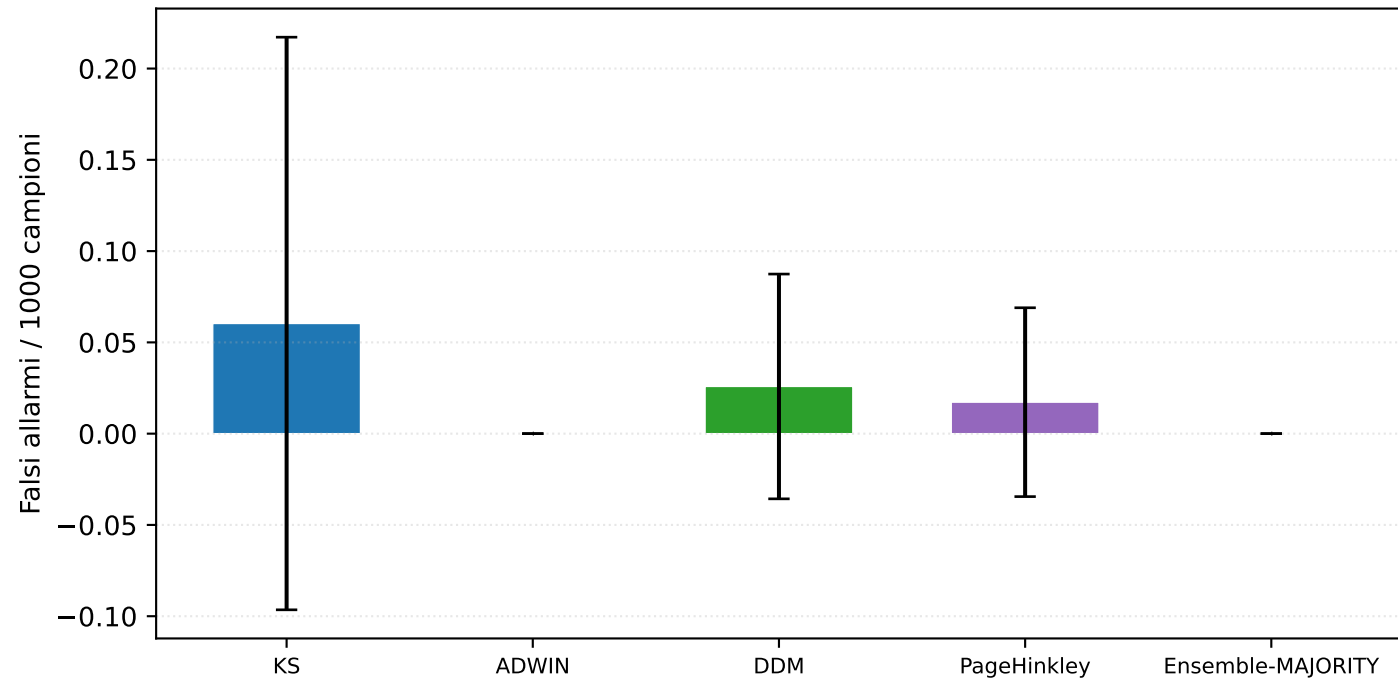
Falsi allarmi su stream stazionario (nessun drift presente)
