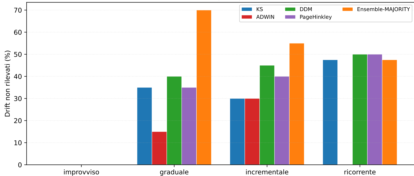
Tasso di mancate rilevazioni per tipo di drift (20 ripetizioni)
