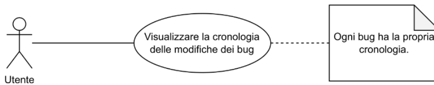
Figura 13: Visualizzazione cronologia modifiche bug use case diagram
