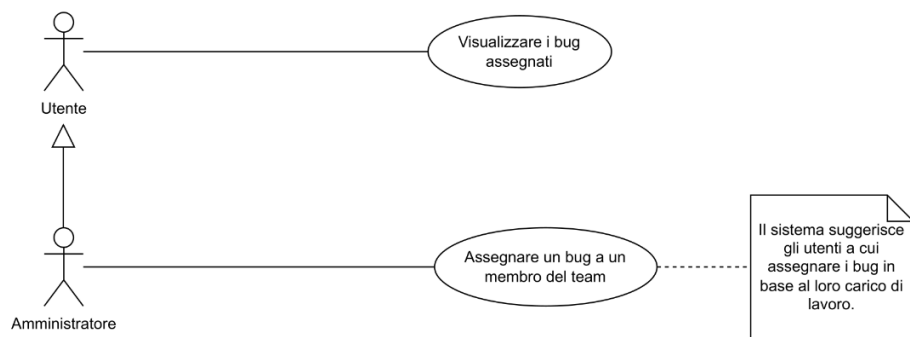
Figura 4: Assegnazione bug use case diagram
