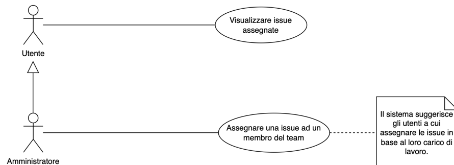
Figura 1.4: Assegnazione issue use case diagram
