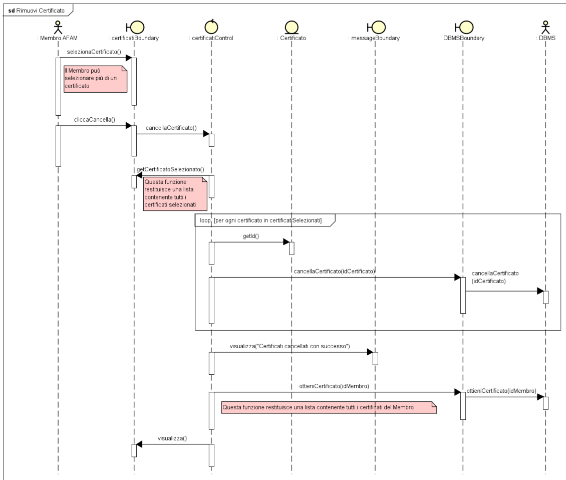
Figure 14: Rimuovi Certificato
