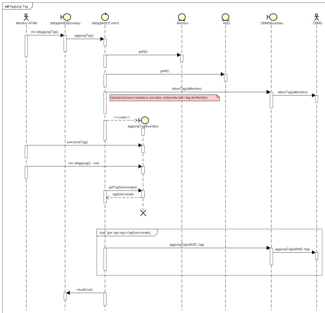
Figure 32: Aggiungi Tag
