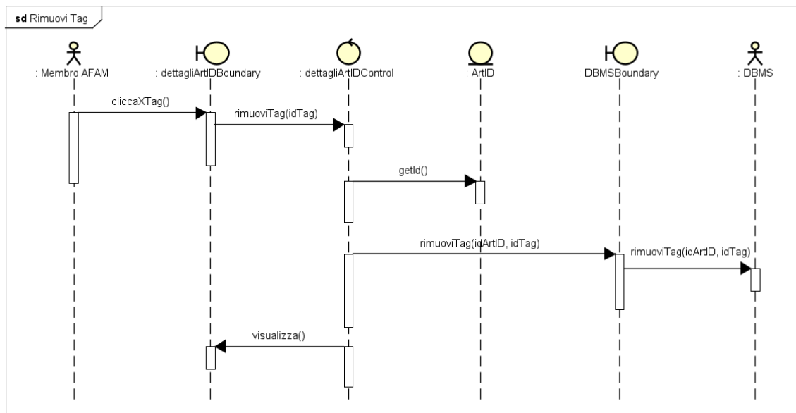
Figure 33: Rimuovi Tag
