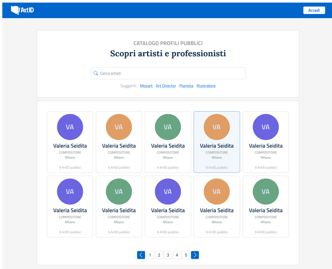
Figure 71: Schermata Esplora
