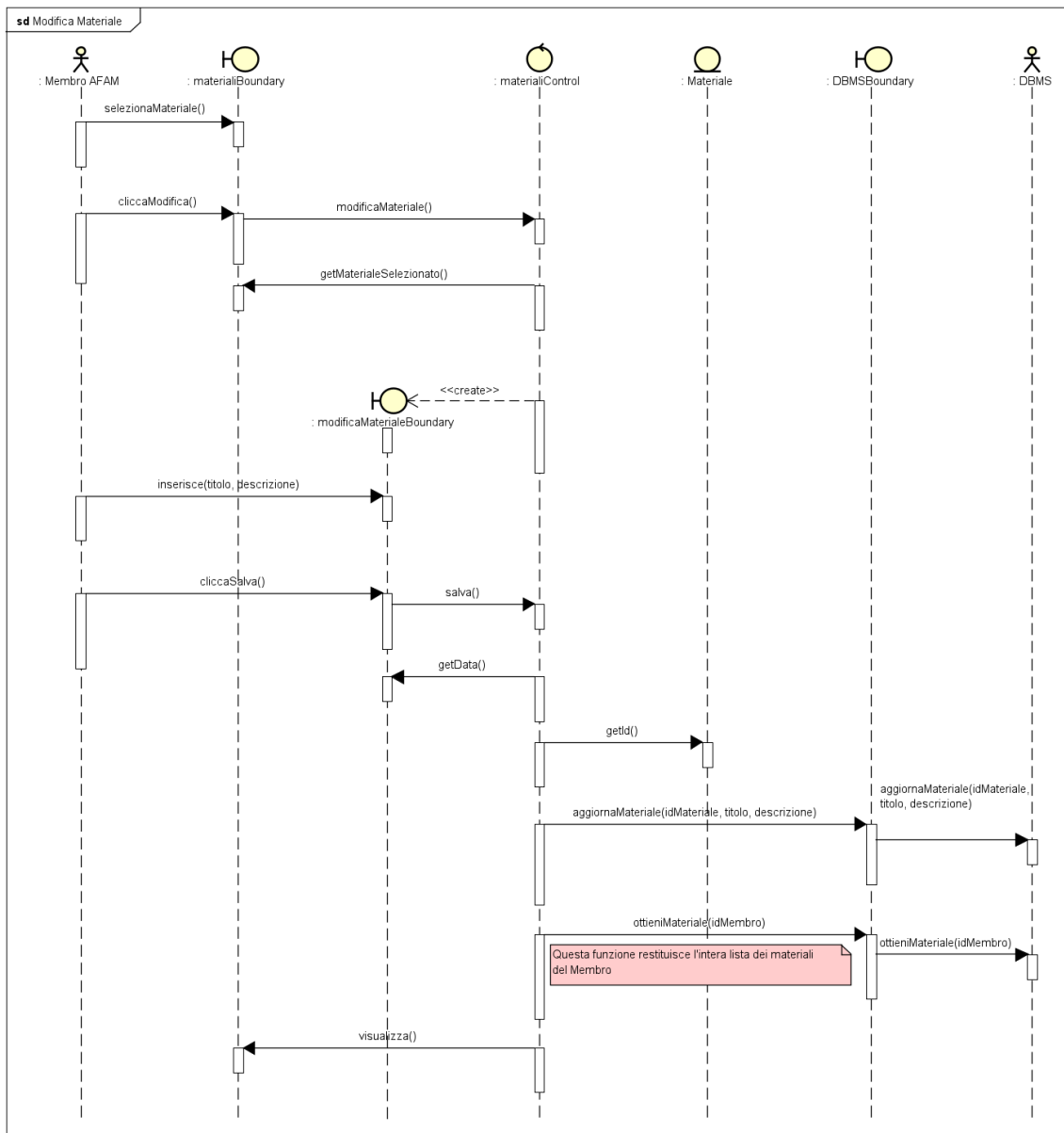
Figure 22: Modifica Materiale
