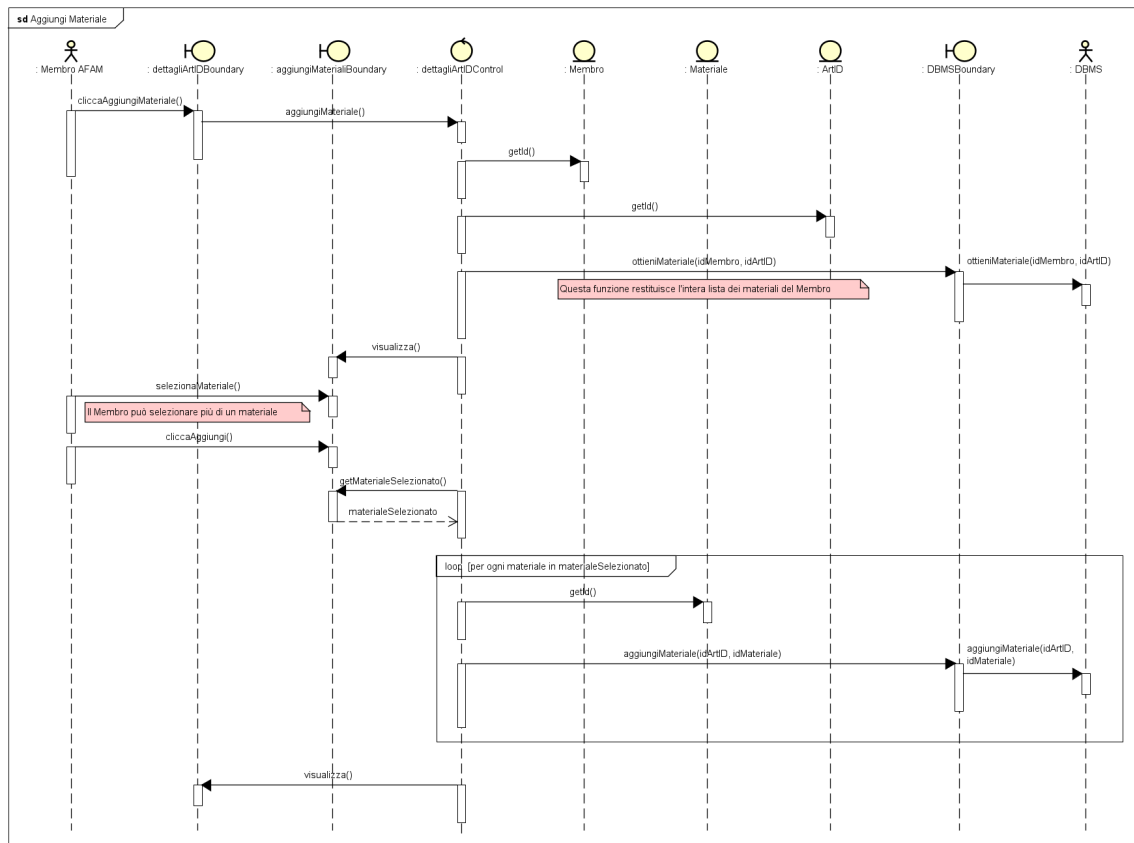
Figure 25: Aggiungi Materiale
