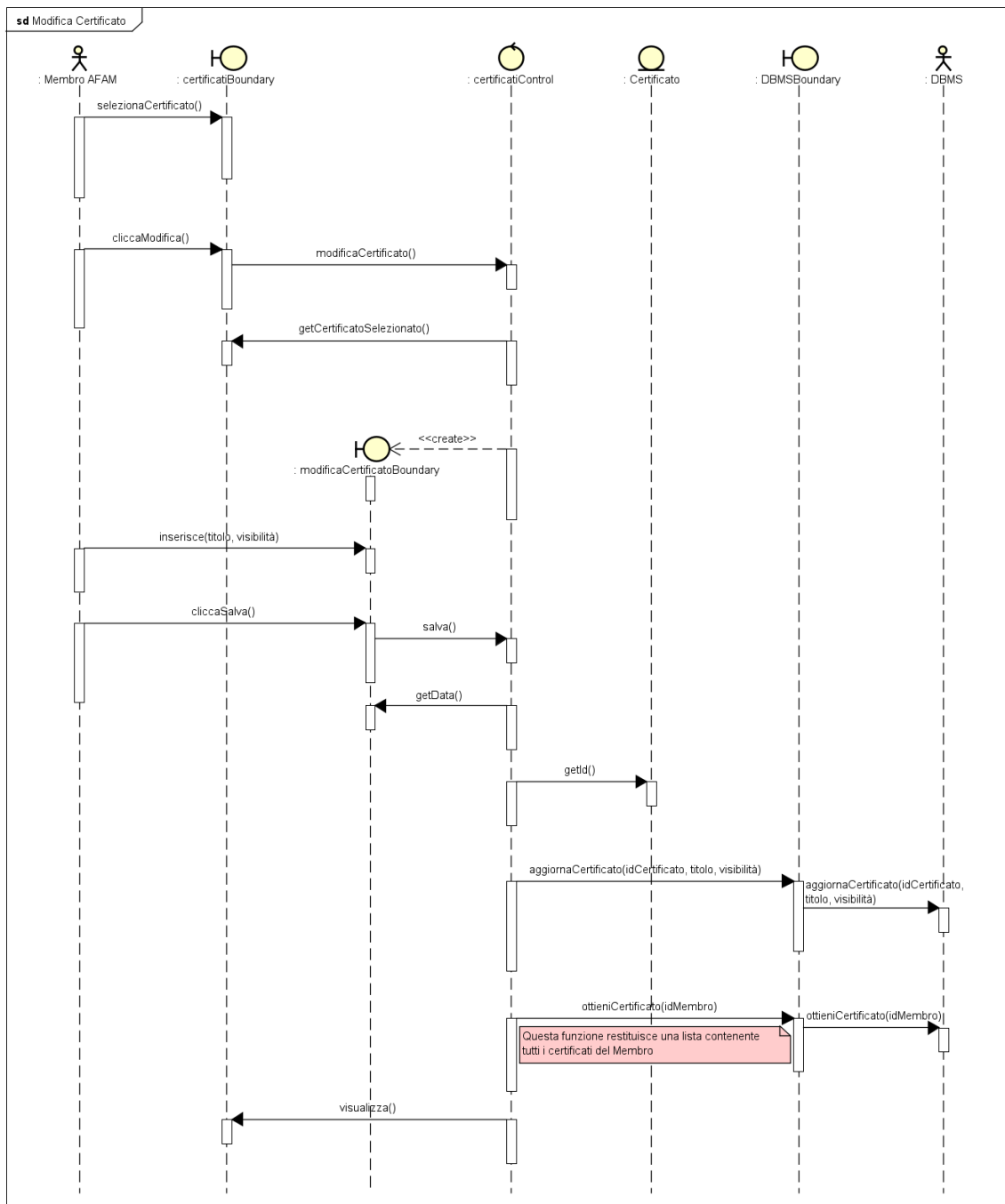
Figure 15: Modifica Certificato
