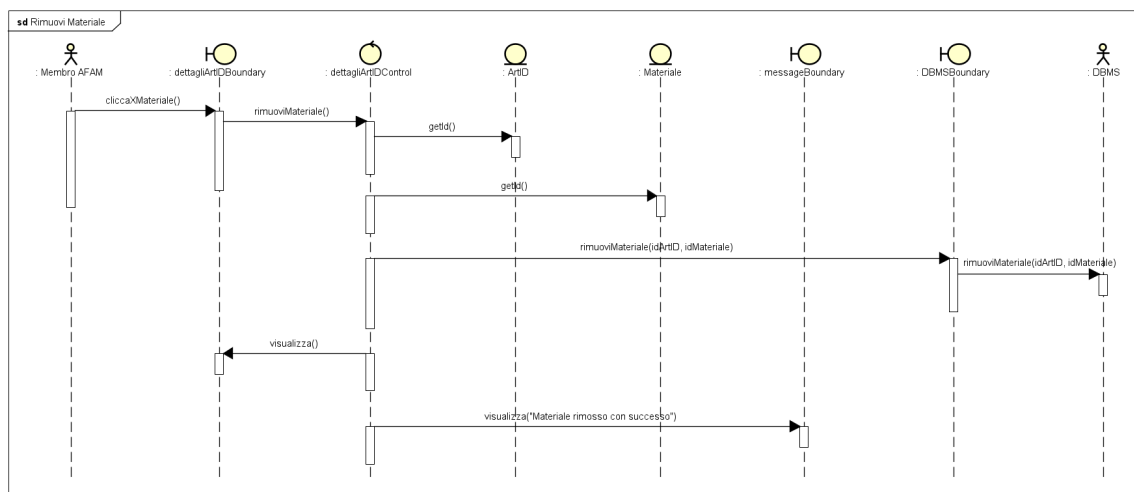
Figure 26: Rimuovi Materiale
