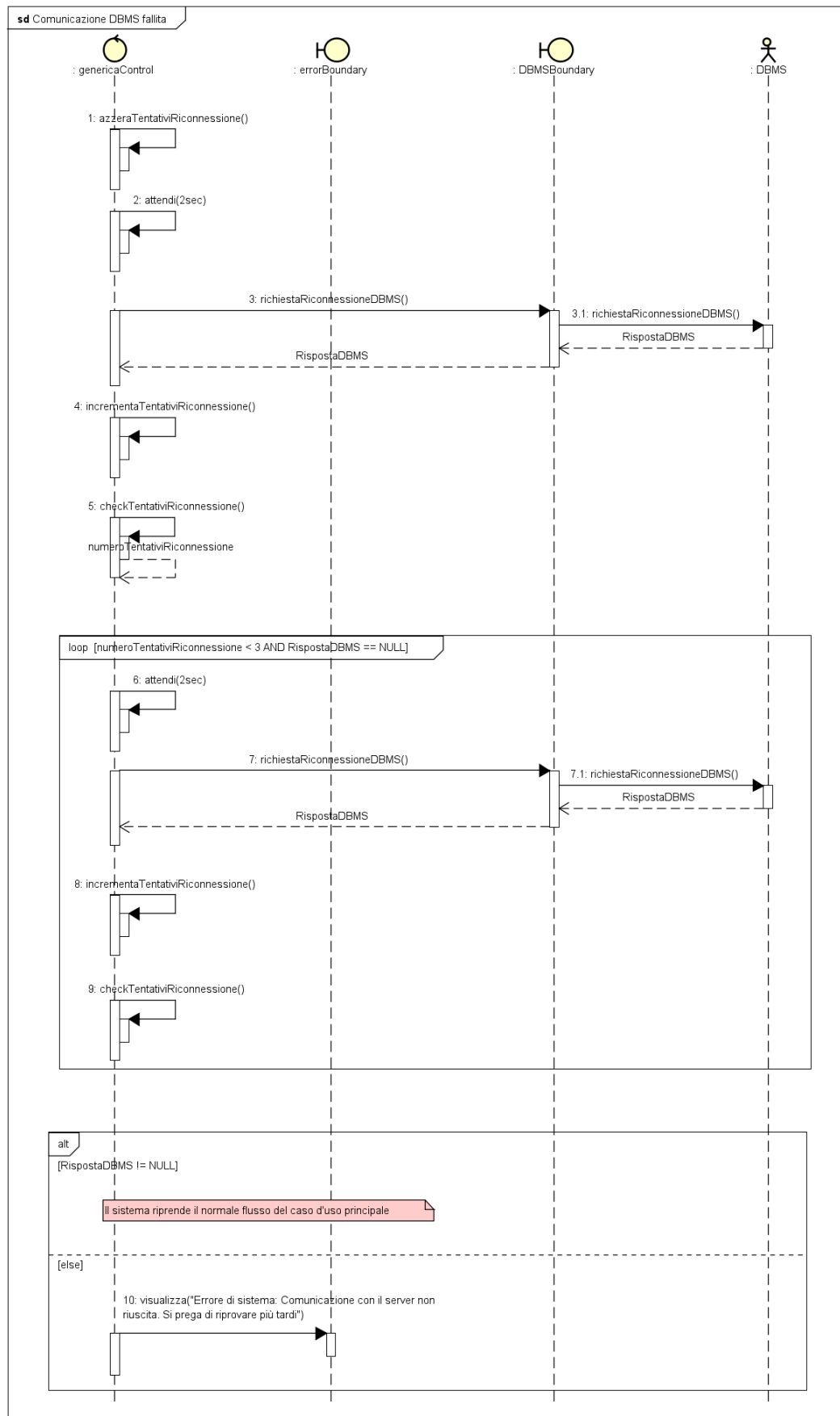
Figure 50: Comunicazione DBMS fallita
