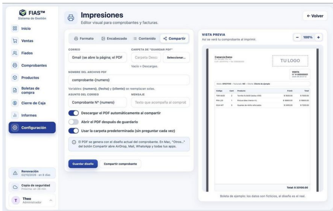
Figura 99 — Impresiones: compartir.
