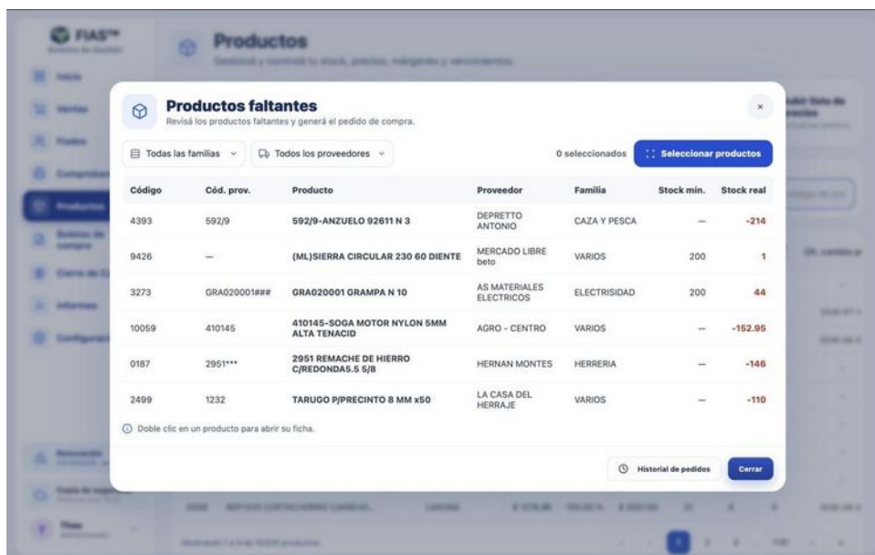
Figura 41 — Productos faltantes.
