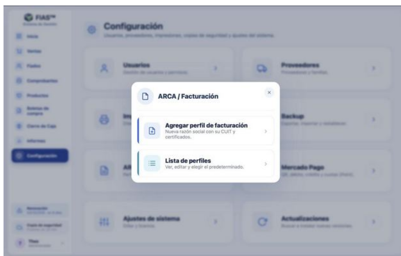
Figura 104 — ARCA / Facturación.
