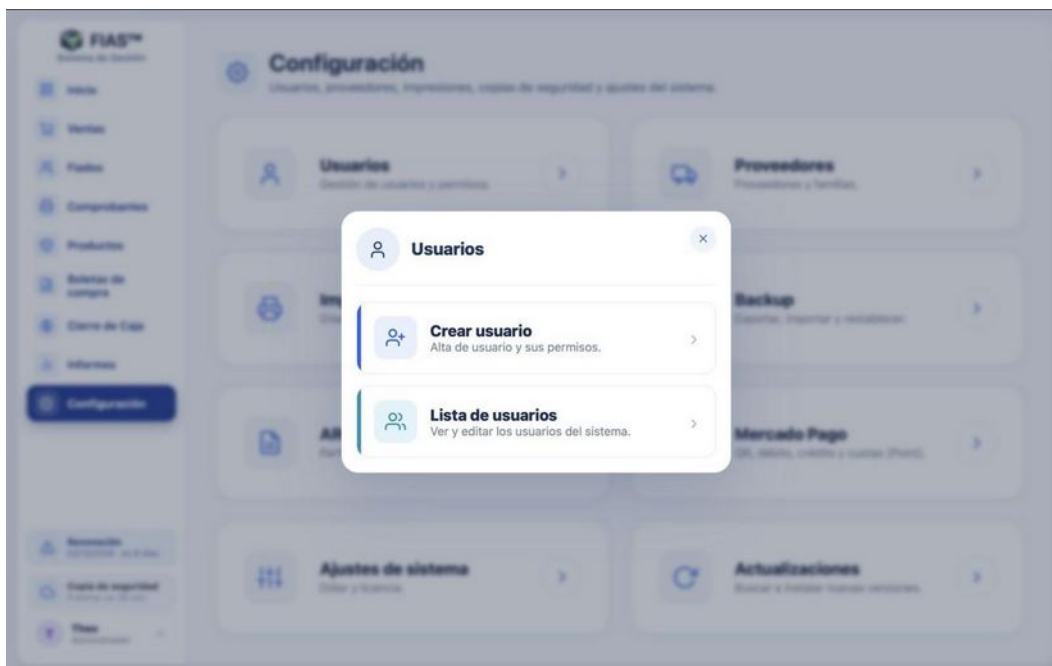
Figura 89 — Usuarios.
