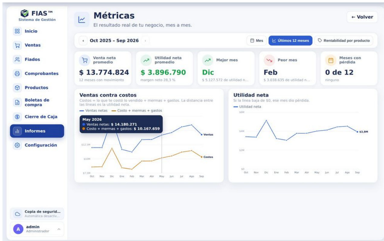
Figura 82 — Últimos 12 meses.
