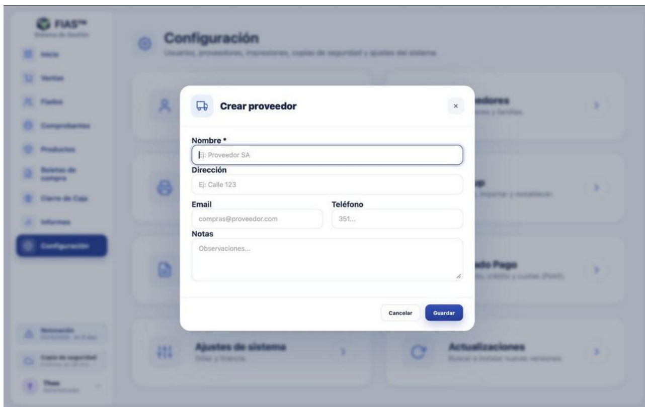
Figura 95 — Crear proveedor.
