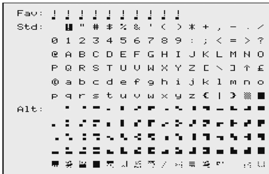
Figure 11: Capture d'écran du mode Palette
