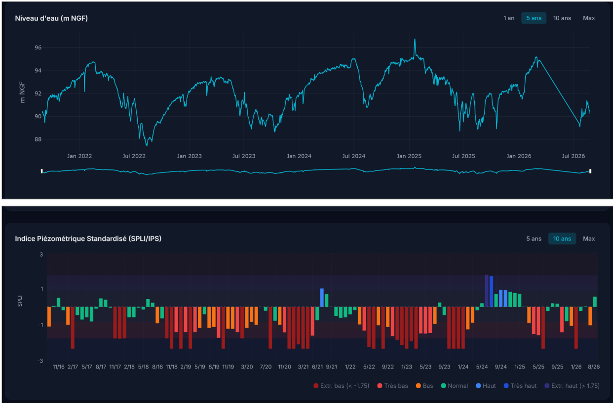
Figure 4.1 – La station de Mur-de-Sologne, en niveau puis en indicateur. En haut la chronique brute sur cinq ans, en mètres NGF : elle situe la mesure dans son unité, mais ne dit pas si le niveau est haut ou bas pour la saison. En bas le même ouvrage sur dix ans en indicateur standardisé mensuel, sur les sept classes. C’est le passage de l’une à l’autre qui rend deux ouvrages comparables, et c’est tout l’objet de ce chapitre.
