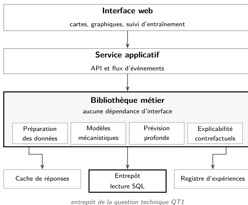
Figure 2 – Architecture de la plateforme. La bibliothèque métier est callable depuis le service web, un script ou un carnet de calcul, sans modification. C’est cette propriété qui rend les méthodes d’explication réutilisables au-delà de l’application qui les héberge.
