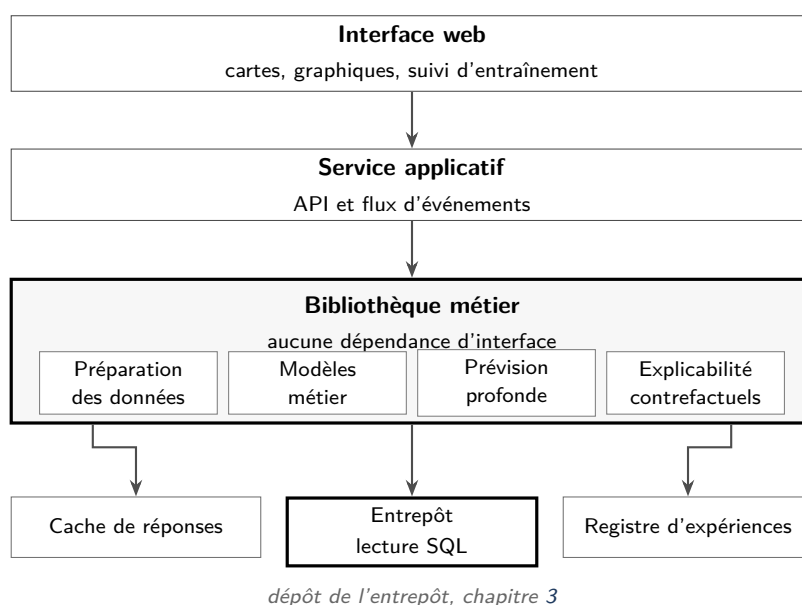
Figure 5.1 – Architecture de la plateforme. La bibliothèque métier est appelable depuis le service web, un script ou un carnet de calcul, sans modification. C'est cette propriété qui rend les développements réutilisables au-delà de l'application.
