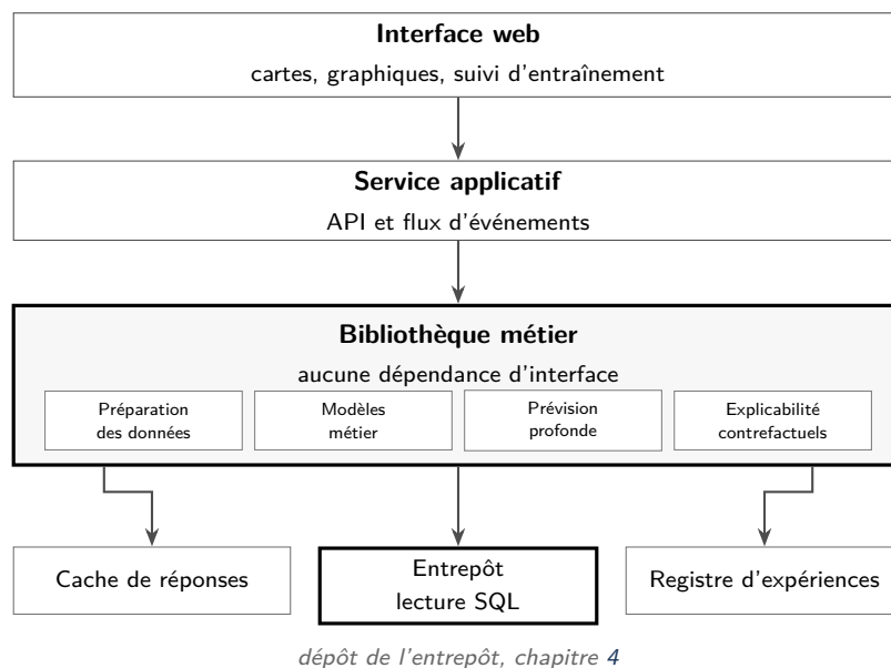
Figure 6.1 – Architecture de la plateforme. La bibliothèque métier est appellable depuis le service web, un script ou un carnet de calcul, sans modification. C'est cette propriété qui rend les développements réutilisables au-delà de l'application.
