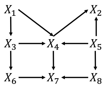
图 2 因果图 \mathcal{H}
