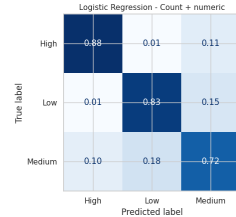
(b) Macierze pomyłek trzech najlepszych modeli.
