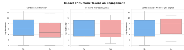
(b) Związek liczb w tekście z logarytmem liczby retweetów.
