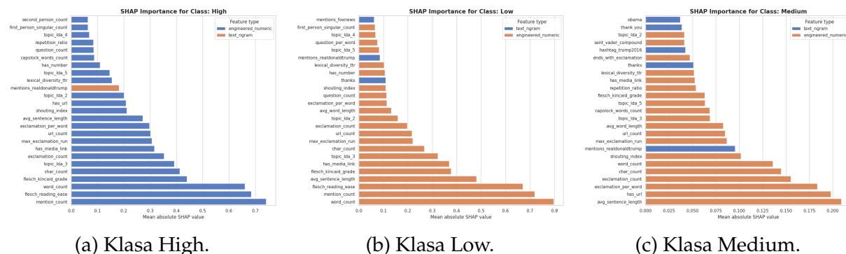
Rysunek 6.2: Najważniejsze cechy |SHAP| dla każdej klasy zainteresowania.
