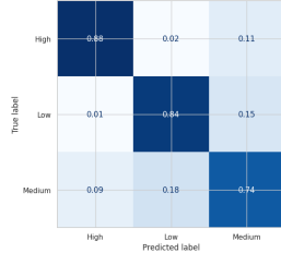
(a) Macierz pomyłek modelu końcowego.
