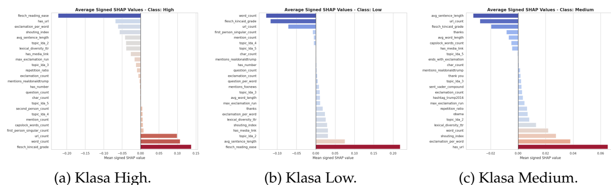
Rysunek 6.3: Najważniejsze cechy SHAP ze znakiem dla każdej klasy zainteresowania.
