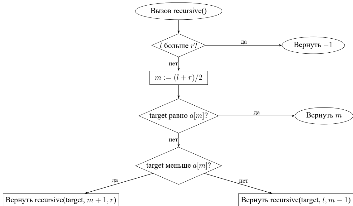
Рисунок 4 – Алгоритм рекурсивного бинарного поиска
