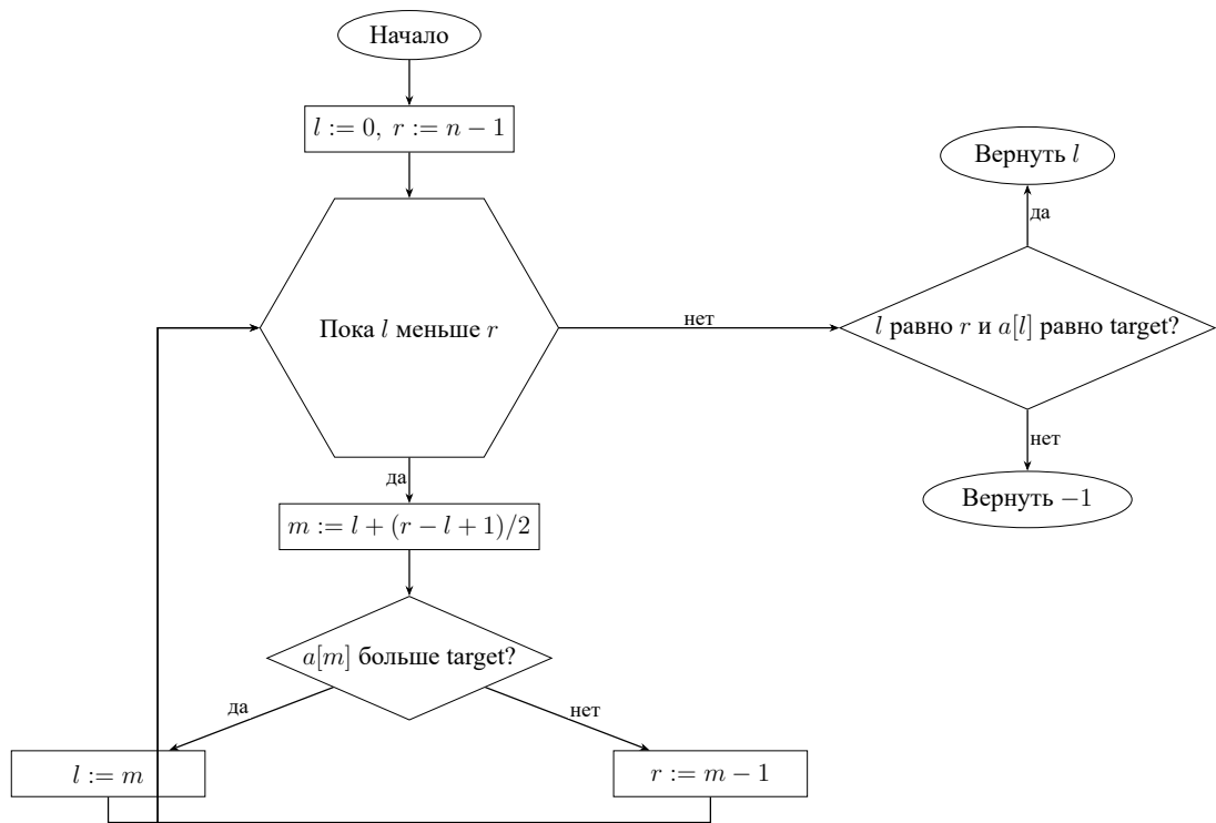
Рисунок 3 – Алгоритм бинарного поиска с одним сравнением
