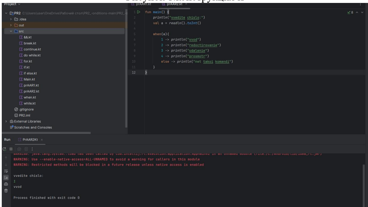
Рисунок 2.конструкция when
