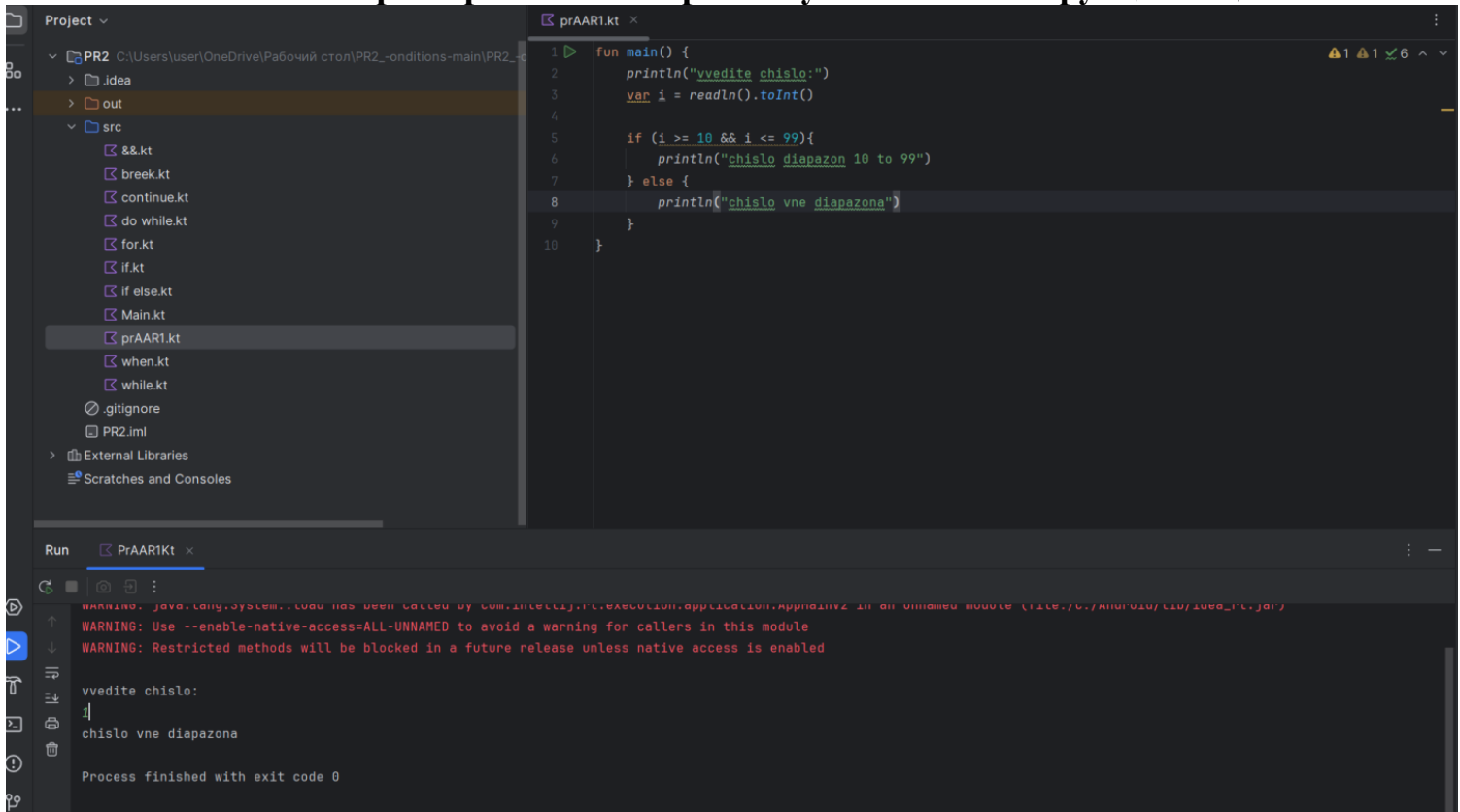
Рисунок 1.конструкция if
