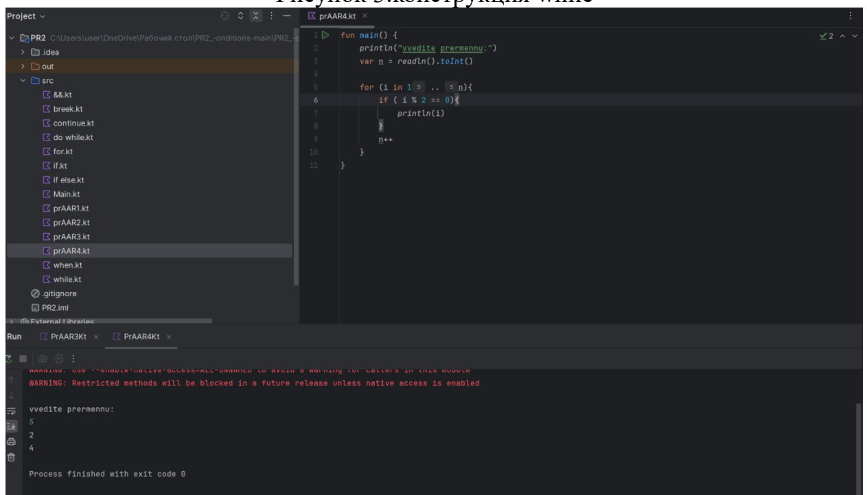
Рисунок 4.конструкция for
