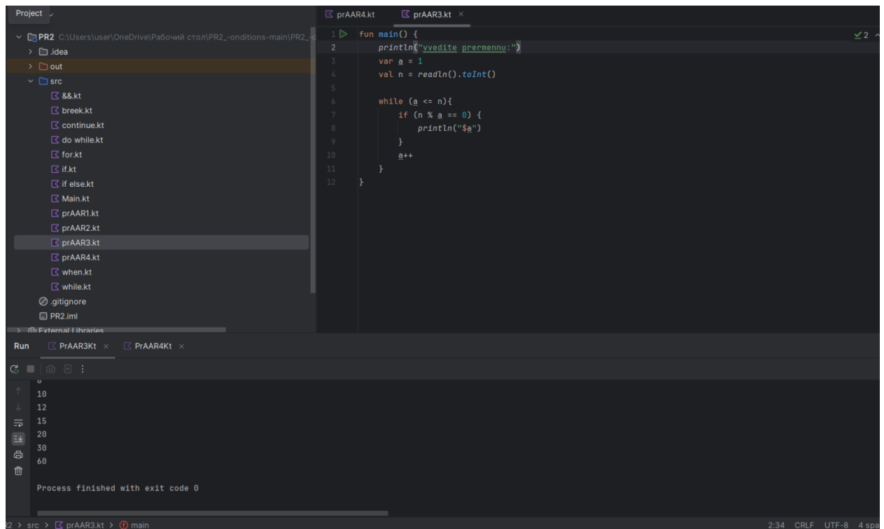
Рисунок 3.конструкция while
