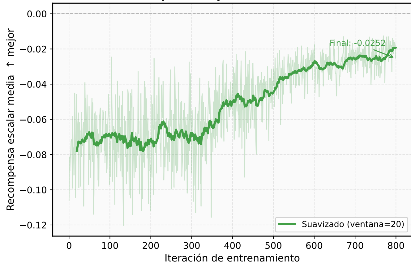
Curva de Aprendizaje — Karate Club (n=34)
