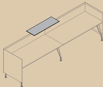
L x W 200x80 / 220x80 / 240x80 H 105 Madera / Lacado / Melamina / Cristal Wood / Lacquered / Melamine / Glass
