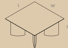
L x W 120x120 / 130x130 / 140x140 / 150x150 / 160x160 H 73
