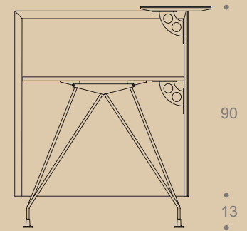
Sección lateral panel suspendido / Lateral section suspended panel Altura total 105cm / Total high 105cm
