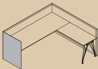
L x W 200x80-180 / 220x80-180 / 240x80-180 H 105 Panel a suelo / Panel to floor Madera / Lacado / Melamina / Cristal Wood / Lacquered / Melamine / Glass
