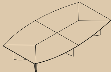
L x W 480x140 / 520x140 / 600x150 H 73 Madera / Lacado Wood / Lacquered
