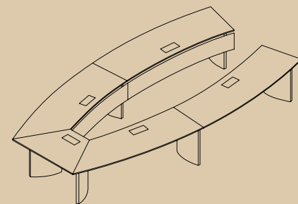
L x W 480x140-220 / 520x140-220 / 600x150 H 73 Madera / Lacado Wood / Lacquered
