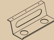
L x W 30 x 7,5 H 9,5 Bandeja apoyo / Support Tray Metal / Metal
