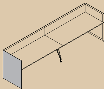
L x W 320x80 / 360x80 / 420x80 H 105 Panel a suelo / Panel to floor Madera / Lacado / Melamina / Cristal Wood / Lacquered / Melamine / Glass
