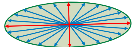
Estirament
