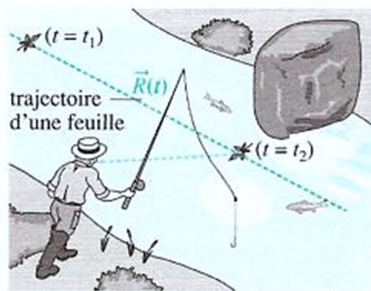
Enfoc Lagrangà
