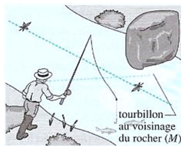
Enfoc Eulerià
