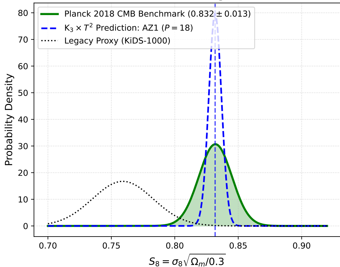
B: S_8 Posterior Alignment
