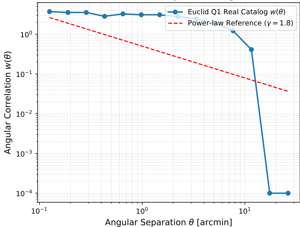
A: Euclid Q1 Galaxy Clustering w(\theta)
