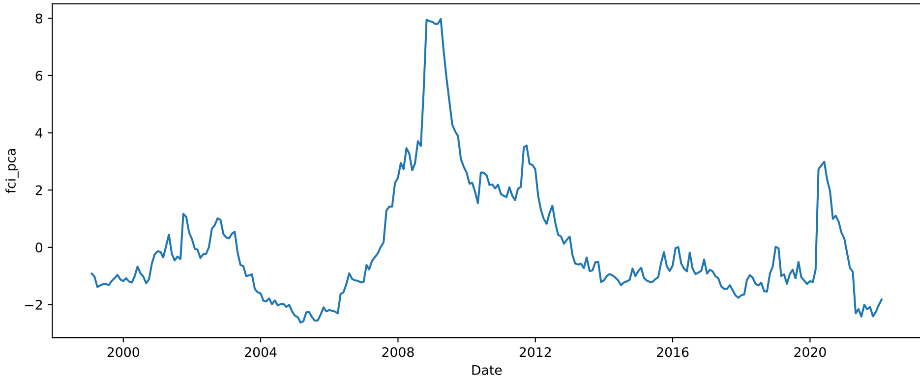
FCI PCA — US
