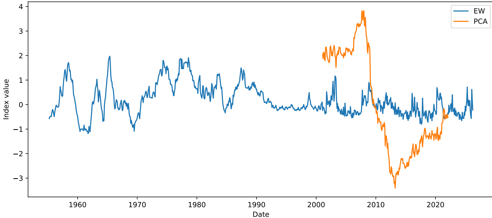
EW vs PCA — ES
