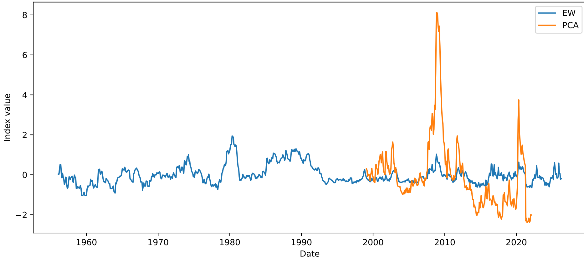
EW vs PCA — UK
