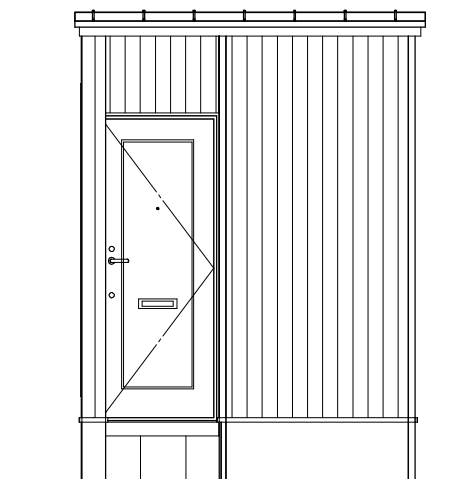
西側 立面図 S:1/50
