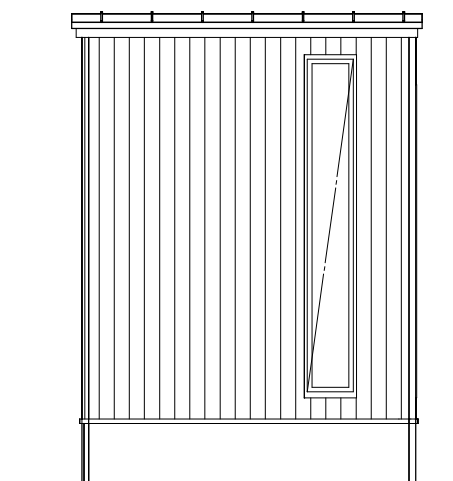
東側 立面図 S:1/50
