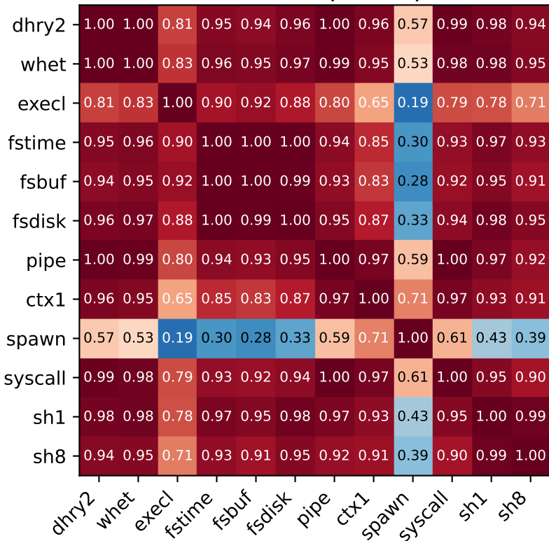
Pearson (n=25)
