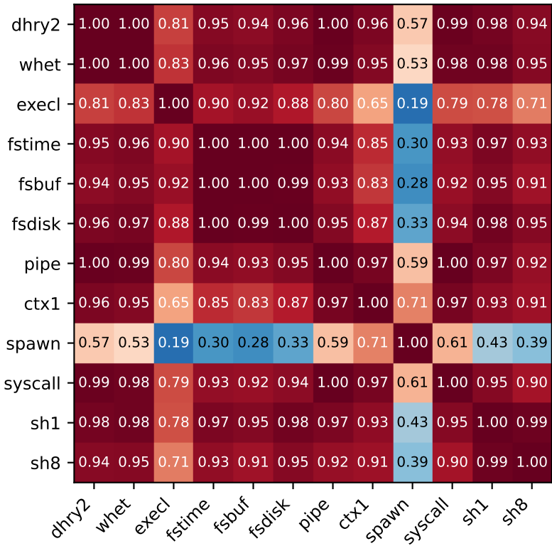
Pearson (n=25)
