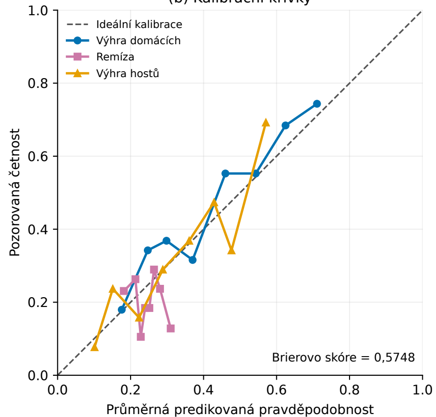
(b) Kalibrační křivky
