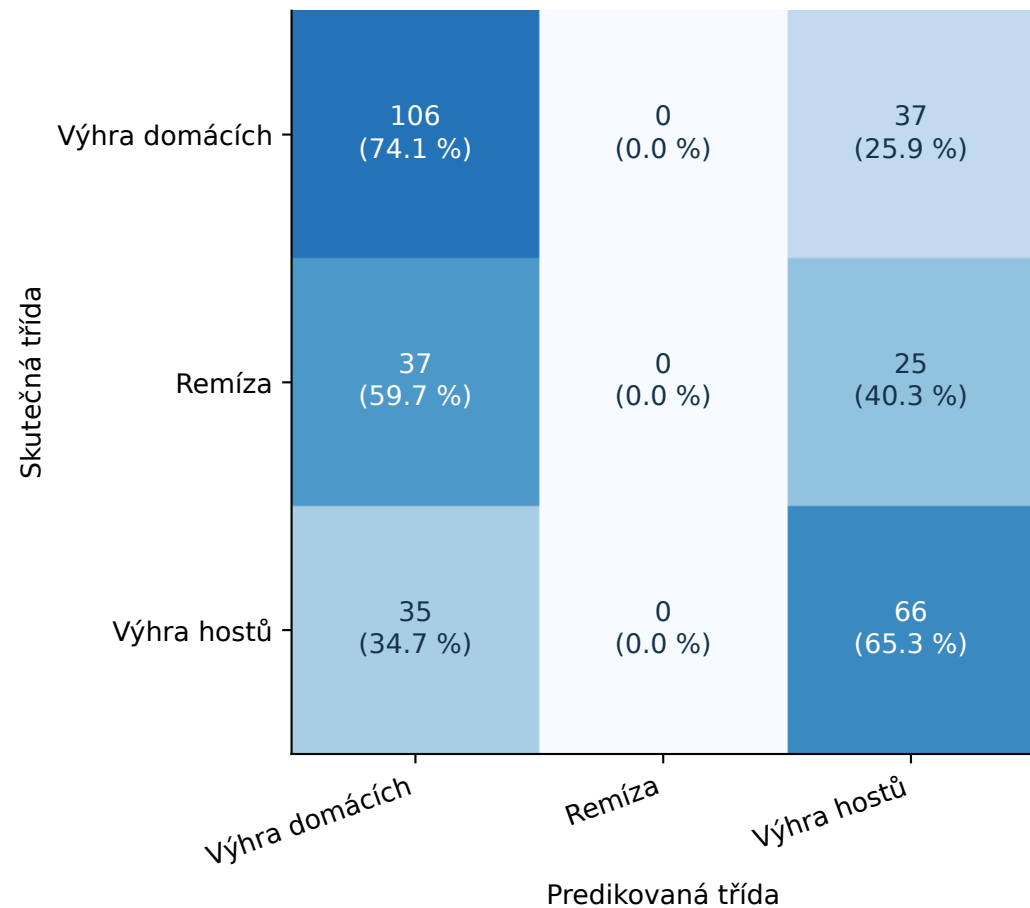
(a) Matice záměn
