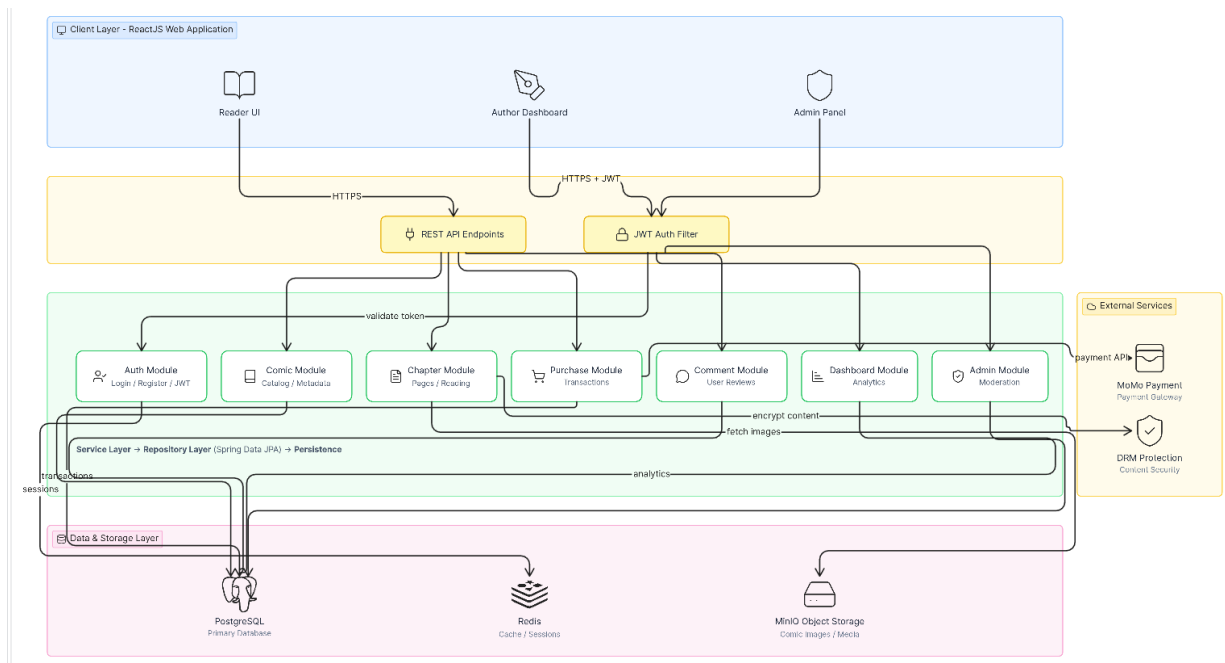
Hình 3.2: Biểu đồ kiến trúc tổng thể của hệ thống
