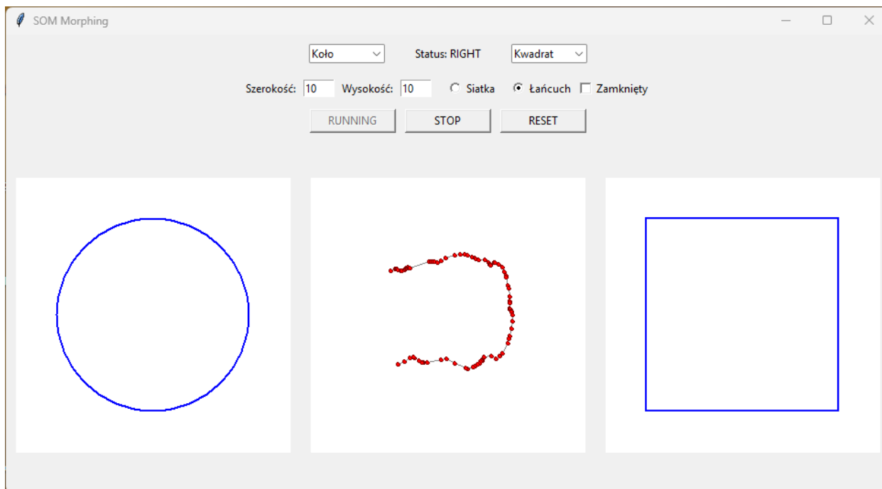
Rys.2 Wizualizacja procesu uczenia sieci SOM w trybie łańcucha[6]
