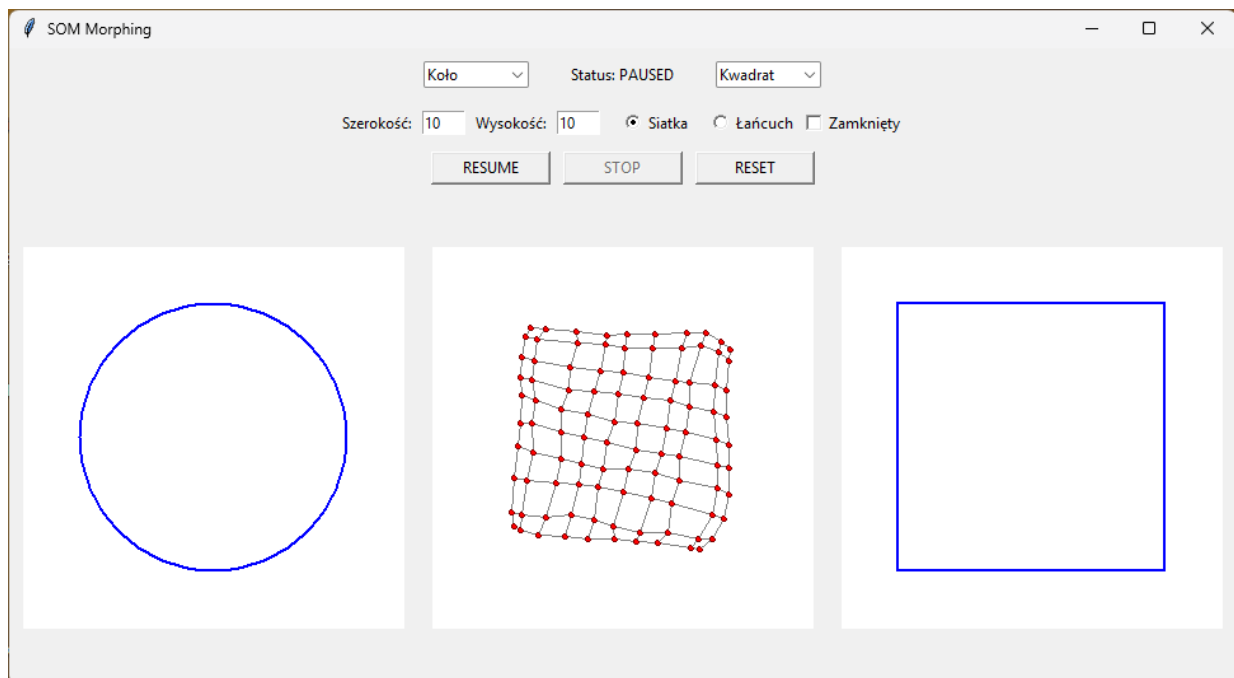
Rys.1 Wizualizacja procesu uczenia sieci SOM w trybie siatki[6]
