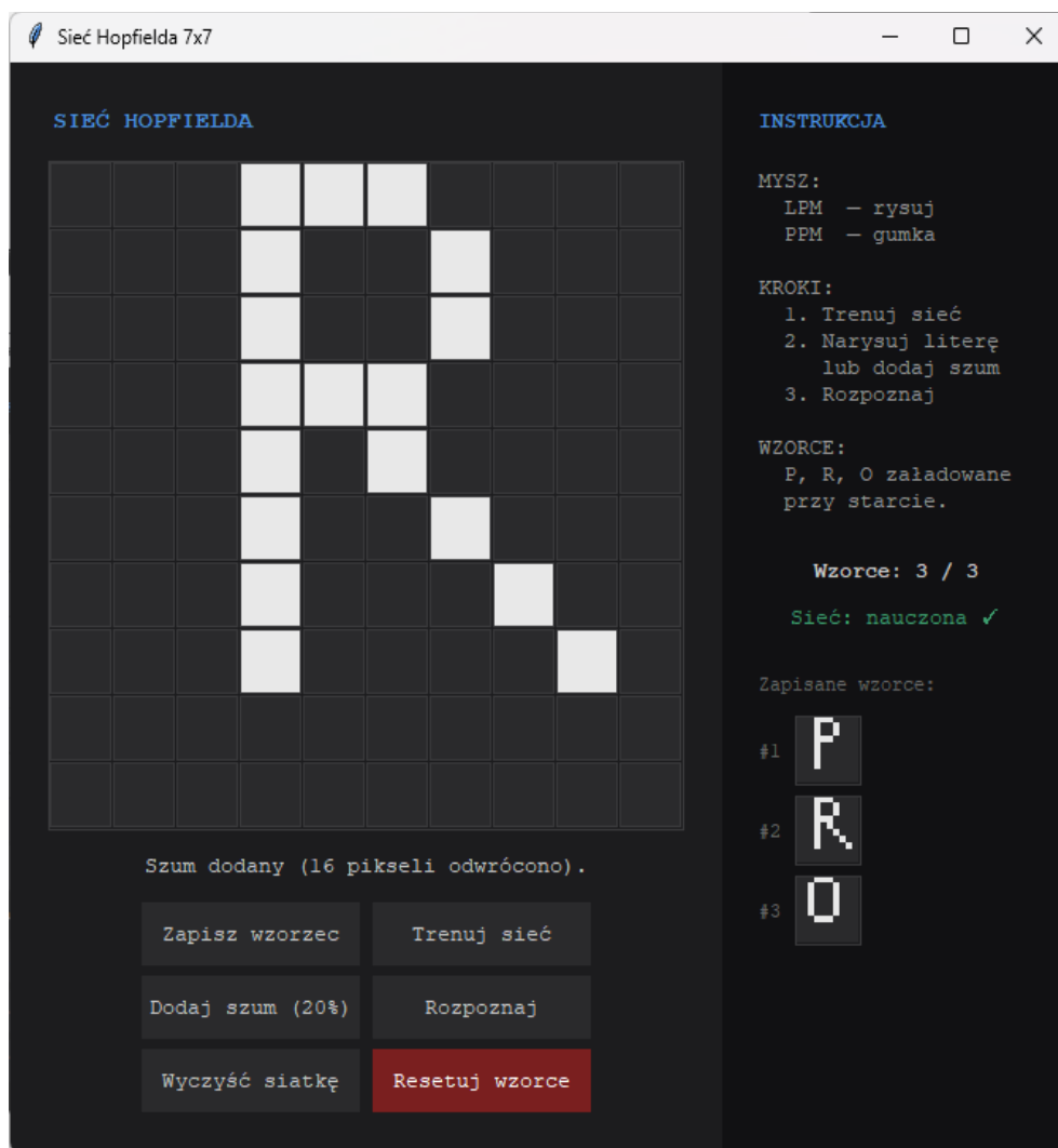
Rys. 4. Wynik działania sieci źródło: Opracowanie własne
