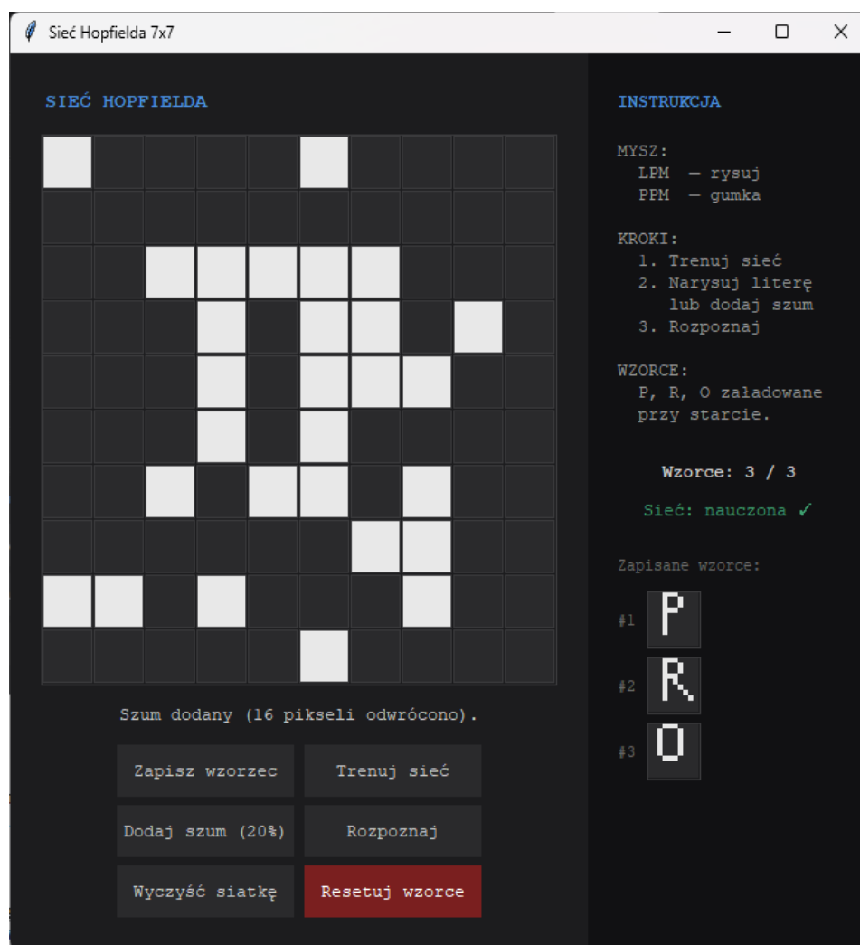
Rys. 3. Zaszumiony wzorzec przed rozpoznaniem źródło: Opracowanie własne
