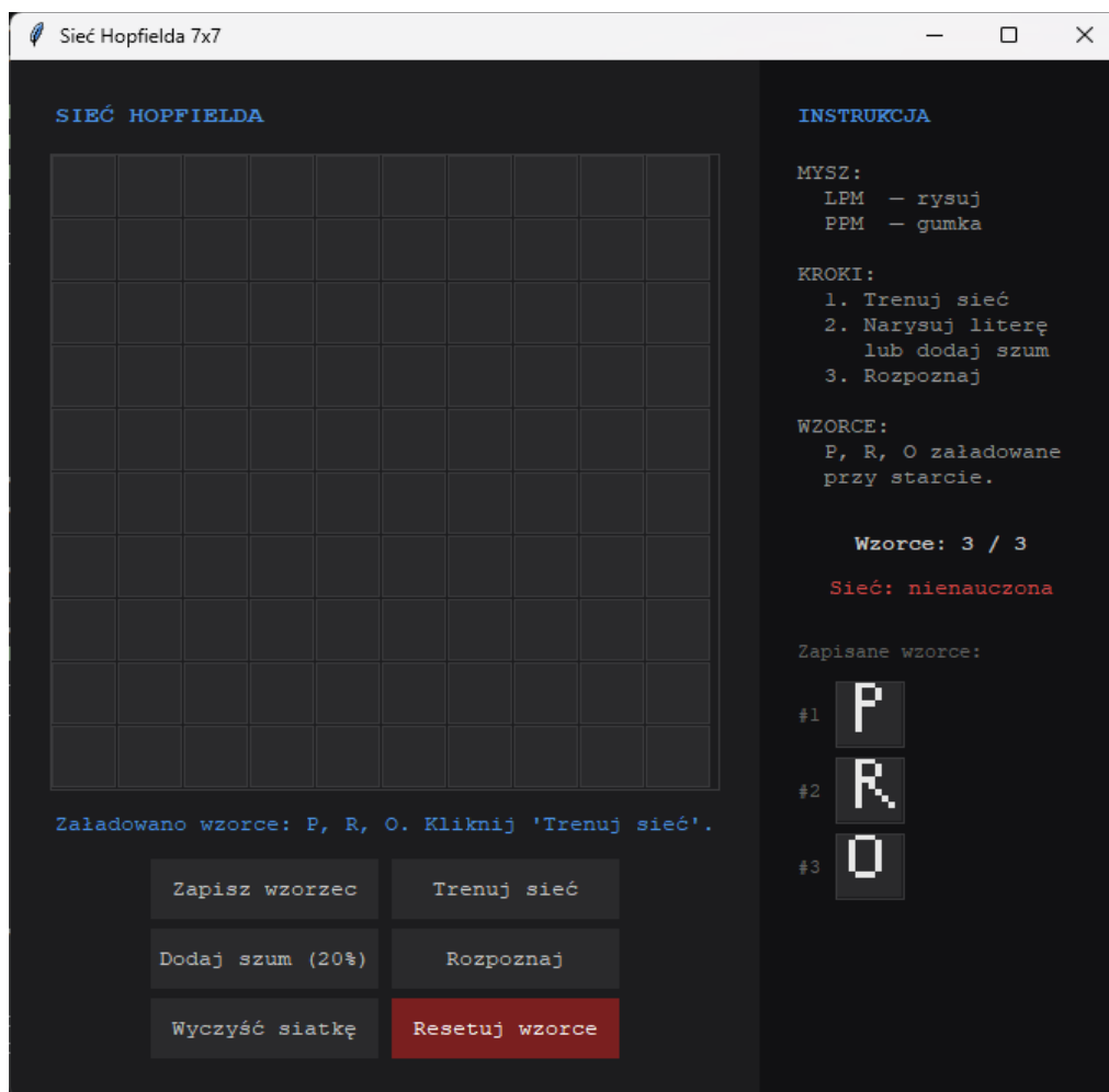
Rys. 2. Interfejs główny programu po uruchomieniu źródło: Opracowanie własne
