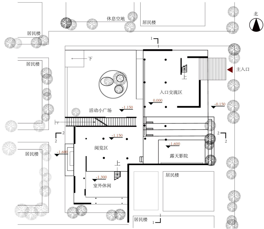
首层平面图 First Floor
