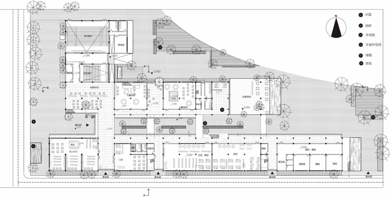
首层平面图 First Floor
