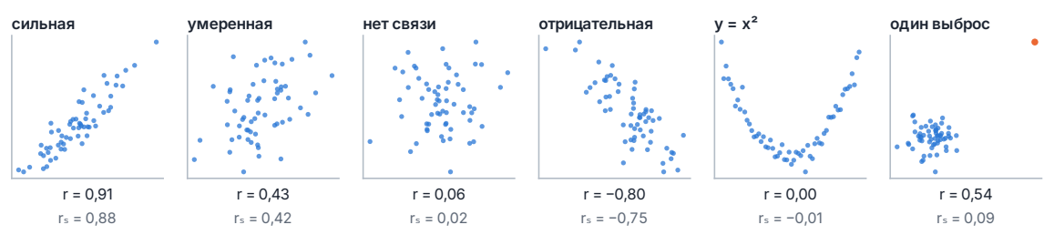
Рис. 3. Коэффициенты Пирсона r и Спирмена r_s на примерах по 60 точек. Парабола: сильная нелинейная связь, но r \approx 0 . Один выброс создаёт r = 0,54 в облаке без связи, а ранговая корреляция остаётся около нуля.
