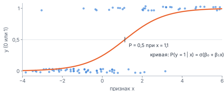
Рис. 17. Логистическая регрессия: точки — наблюдения 0 и 1 (сдвинуты по вертикали, чтобы не сливались), кривая — оцененная вероятность P(y = 1 | x) .
