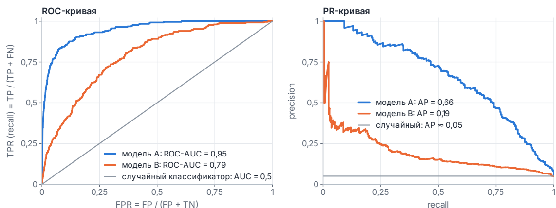
Рис. 21. ROC- и PR-кривые двух моделей на 5 000 объектах, из которых 5% положительные. ROC-кривая модели В выглядит прилично, но PR-кривая показывает низкую precision.
