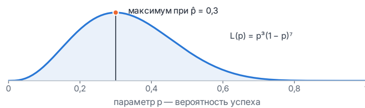
Рис. 8. Функция правдоподобия для 3 успехов в 10 испытаниях. Максимум — в точке \hat{p} = 0,3 .
