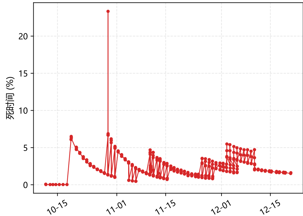
HPGe 死时间随测量时间变化
