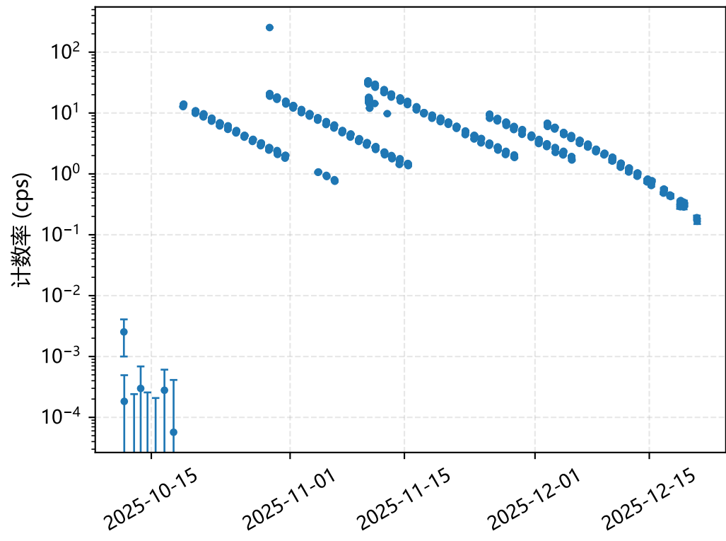
747keV 峰计数率
