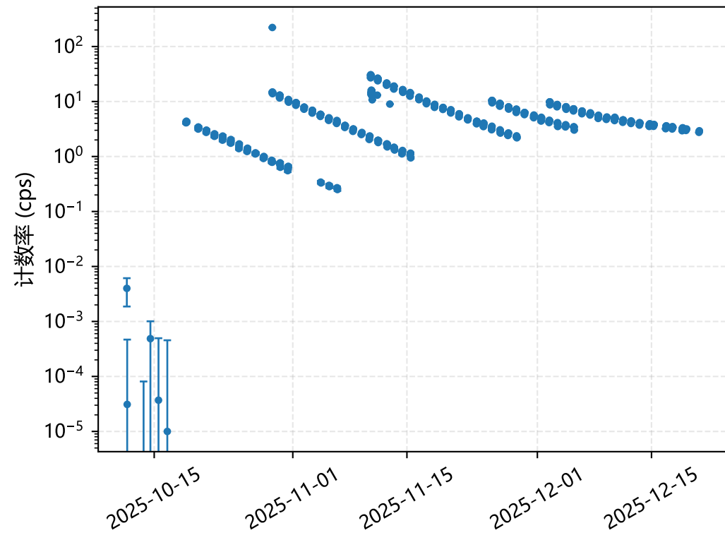
633keV 峰计数率
