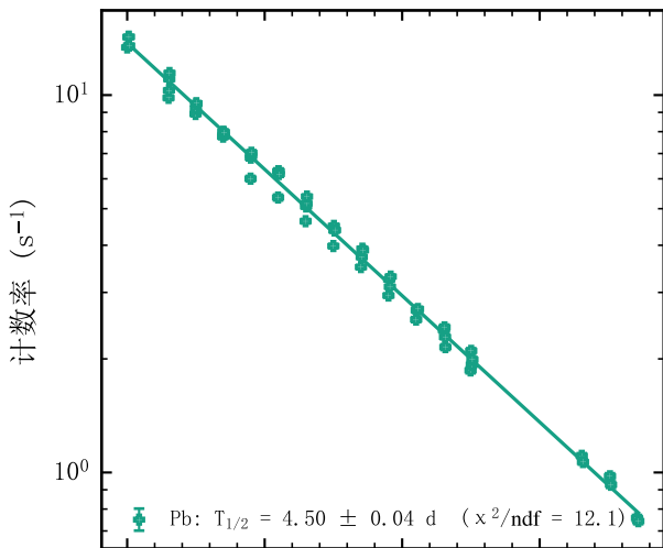
^{146}\text{Eu} 衰变曲线 (747keV)
