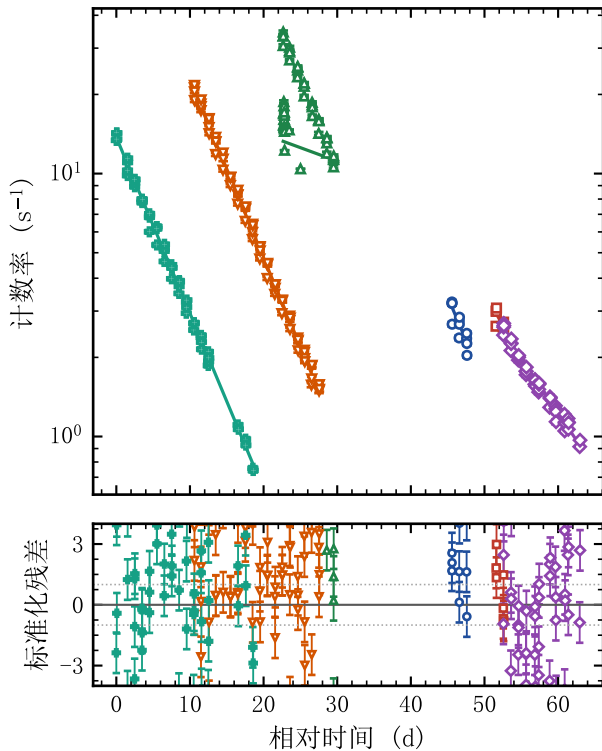
^{146}\text{Eu} 衰变曲线 (747keV)
