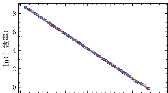
第 1 组 (靶室 1) — 633keV
