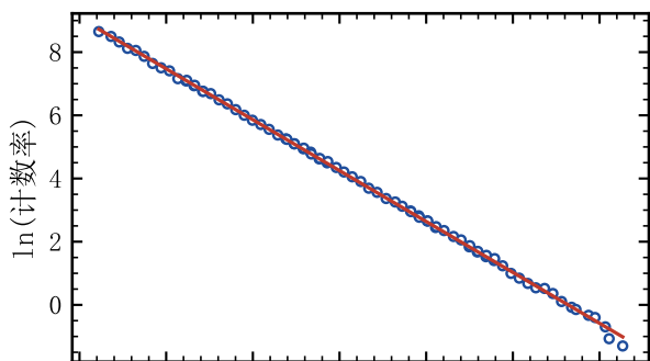
第 2 组 (靶室 2) — 633keV
