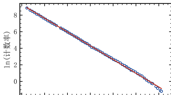
第 3 组 (靶室 3) — 747keV
