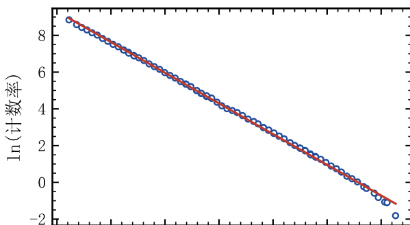
第 2 组 (靶室 2) — 747keV
