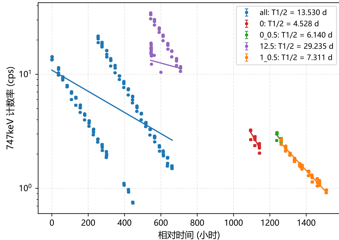
146Eu 衰变曲线
