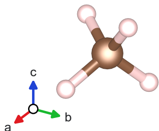
(j) CH 4 0D, molecule
