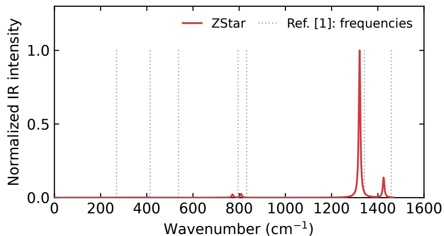
(a) BN(6,0) nanotube | IR
