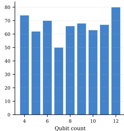
VQC
