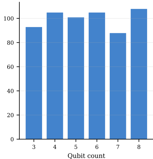
Deutsch-Jozsa
