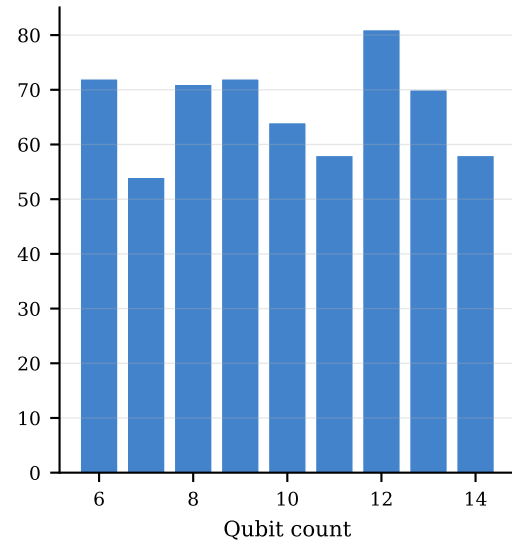
QAOA
