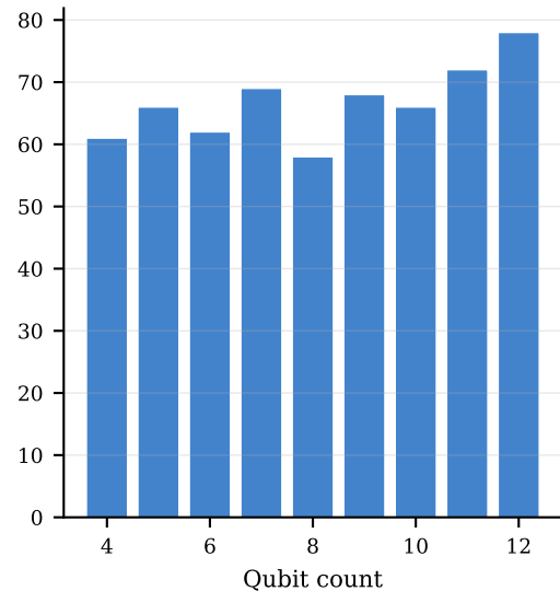
QFT
