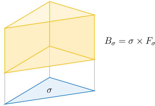
Рис. 3: Блок тоск-расслоения над треугольником \sigma ; слой F_\sigma условно изображён отрезком.
